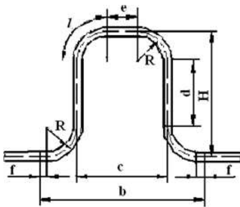
Рис. 25. Π-образный компенсатор
