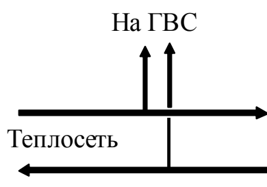
Рис. 3. Схема подключения системы ГВС к открытой тепловой сети
