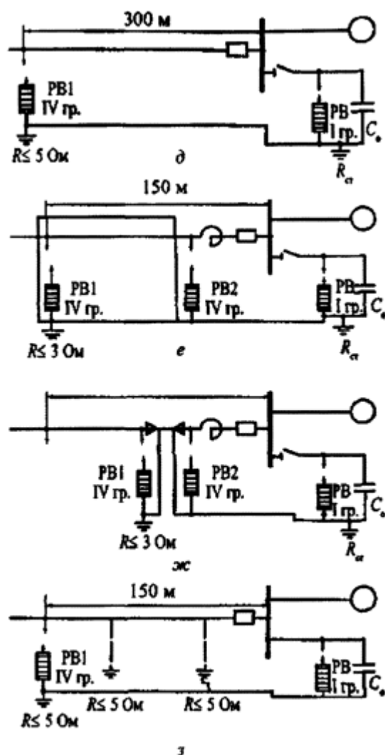
Рис. 4.2.20. Схемы защиты вращающихся электрических машин от грозowych перенапряжений
