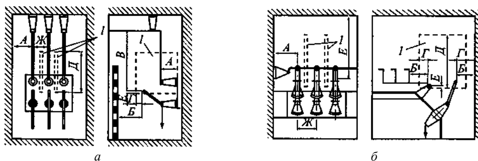
Рис. 4.2.2. Установка разъединителя (отделителя): а - вертикальная; б — наклонная; 1 — изолирующие перегородки
