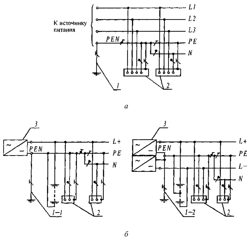
Рис. 1.7.3. Система TN-C-S переменного ( a ) и постоянного ( б ) тока. Нулевой защитный и нулевой рабочий проводники совмещены в одном проводнике в части системы: 1 — заземлитель нейтрали источника переменного тока; 1-1 - заземлитель вывода источника постоянного тока; 1-2 - заземлитель средней точки источника постоянного тока; 2 - открытые проводящие части, 3 - источник питания
